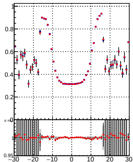
Fake rate vs d —•— DQM TT mkFit —•— DQM TT mkFit BDT
