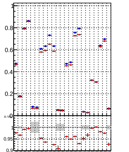
Fake rate vs. —●— DQM TT mkFit —●— DQM TT mkFit BDT
