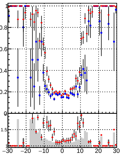
Fake rate vs d —●— DQM TT mkFit —●— DQM TT mkFit BDT
