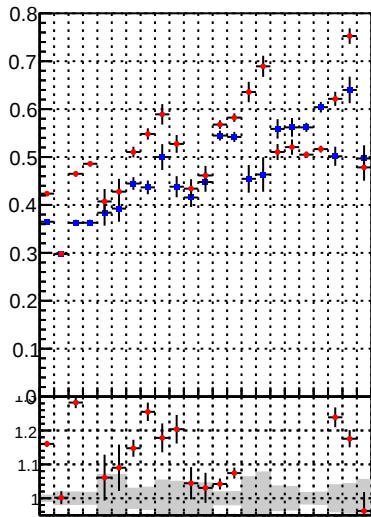
Fake rate vs. —●— DQM TT_mkFit —●— DQM TT_mkFit_BDT
