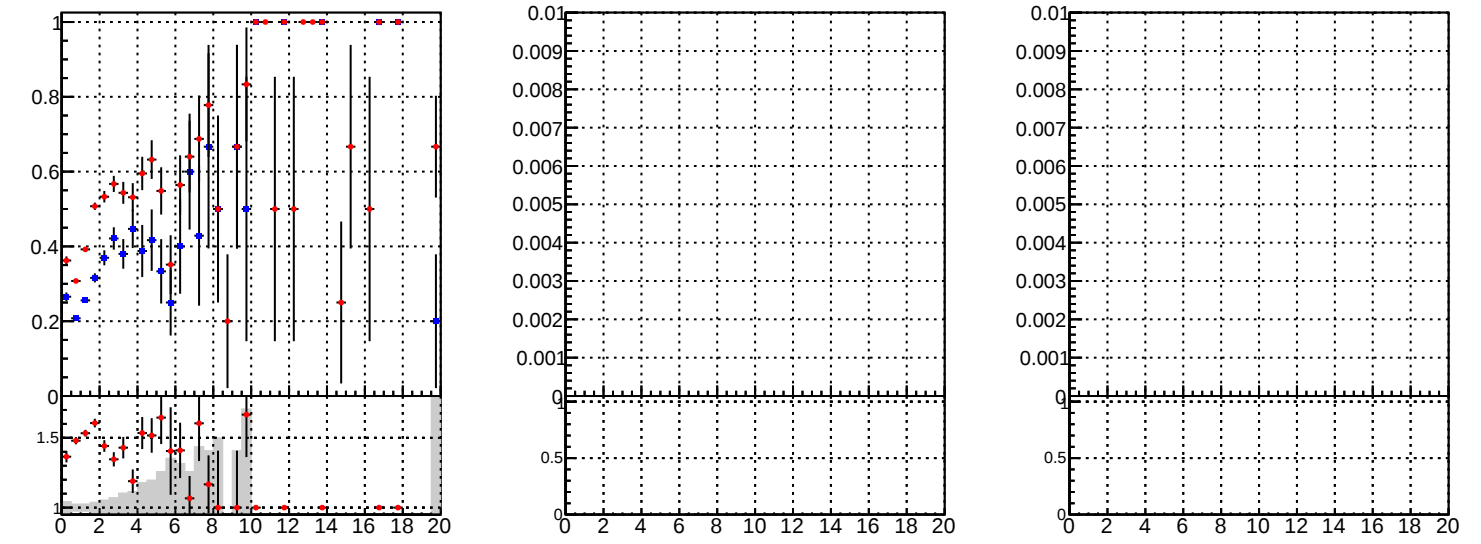
Fake rate vs. —●— DQM TT mkFit —●— DQM TT mkFit BDT
