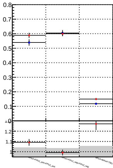
Fake rate vs. —●— DQM TT mkFit —●— DQM TT mkFit BDT
