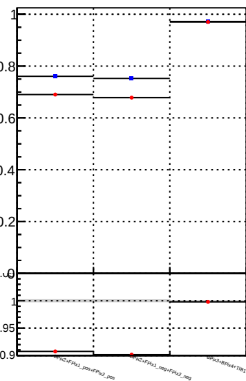
Fake rate vs. DQM TT mkFit DQM TT mkFit BDT
