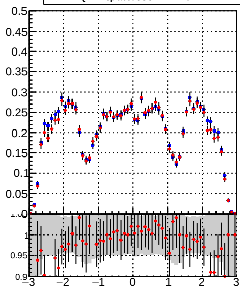
■ DQM_DisplacedSUSY_mkFit_ ■ DQM_DisplacedSUSY_mkFit_BDT_
