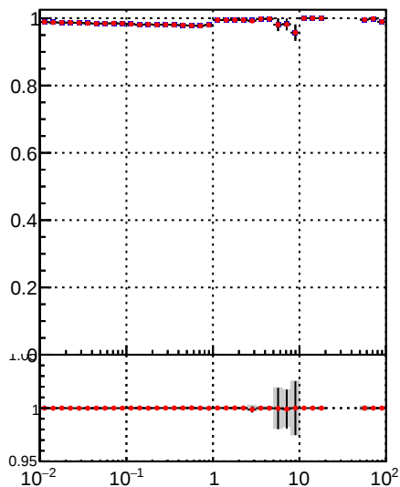
—•— DQM_DisplacedSUSY_mkFit_ —•— DQM_DisplacedSUSY_mkFit_BDT_
