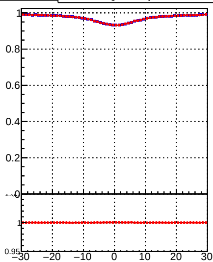
—•— DQM_DisplacedSUSY_mkFit_ —•— DQM_DisplacedSUSY_mkFit_BDT_
