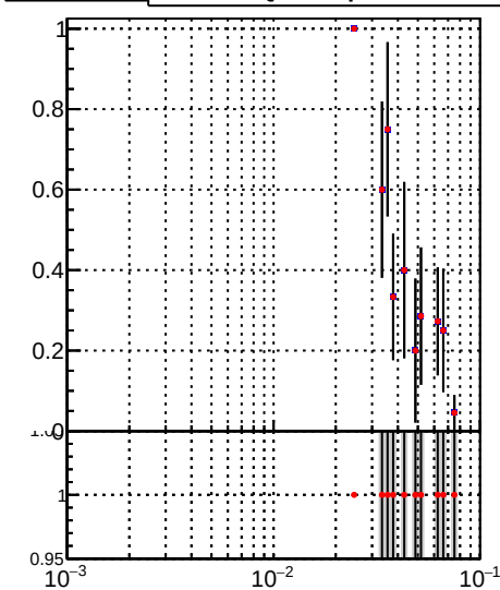
—•— DQM_DisplacedSUSY_mkFit_ —•— DQM_DisplacedSUSY_mkFit_BDT_
