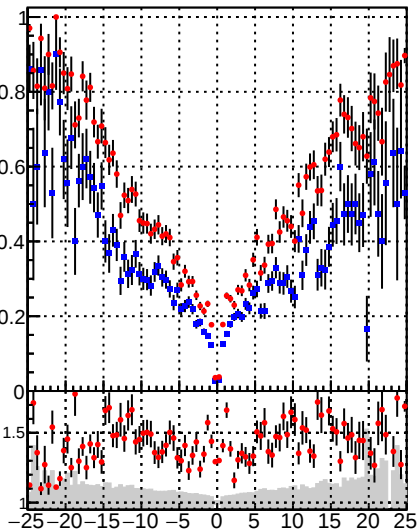
Fake rate vs \Delta y
