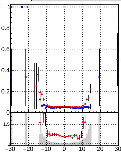
■ DQM_DisplacedSUSY_mkFit_ ● DQM_DisplacedSUSY_mkFit_BDT_
