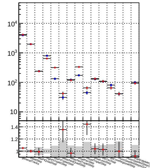
Number DQM_DisplacedSUSY_mkFit_BDT_ 1 0.000000 2 0.000000 3 0.000000 4 0.000000 5 0.000000 6 0.000000 7 0.000000 8 0.000000 9 0.000000 10 0.000000 11 0.000000 12 0.000000 13 0.000000 14 0.000000 15 0.000000 16 0.000000 17 0.000000 18 0.000000 19 0.000000 20 0.000000 21 0.000000 22 0.000000 23 0.000000 24 0.000000 25 0.000000 26 0.000000 27 0.000000 28 0.000000 29 0.000000 30 0.000000 31 0.000000 32 0.000000 33 0.000000 34 0.000000 35 0.000000 36 0.000000 37 0.000000 38 0.000000 39 0.000000 40 0.000000 41 0.000000 42 0.000000 43 0.000000 44 0.000000 45 0.000000 46 0.000000 47 0.000000 48 0.000000 49 0.000000 50 0.000000 51 0.000000 52 0.000000 53 0.000000 54 0.000000 55 0.000000 56 0.000000 57 0.000000 58 0.000000 59 0.000000 60 0.000000 61 0.000000 62 0.000000 63 0.000000 64 0.000000 65 0.000000 66 0.000000 67 0.000000 68 0.000000 69 0.000000 70 0.000000 71 0.000000 72 0.000000 73 0.000000 74 0.000000 75 0.000000 76 0.000000 77 0.000000 78 0.000000 79 0.000000 80 0.000000 81 0.000000 82 0.000000 83 0.000000 84 0.000000 85 0.000000 86 0.000000 87 0.000000 88 0.000000 89 0.000000 90 0.000000 91 0.000000 92 0.000000 93 0.000000 94 0.000000 95 0.000000 96 0.000000 97 0.000000 98 0.000000 99 0.000000 100 0.000000
