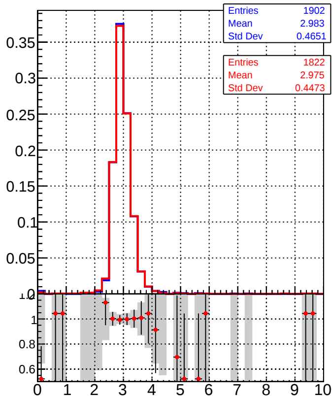
dE/dx estimator 2
