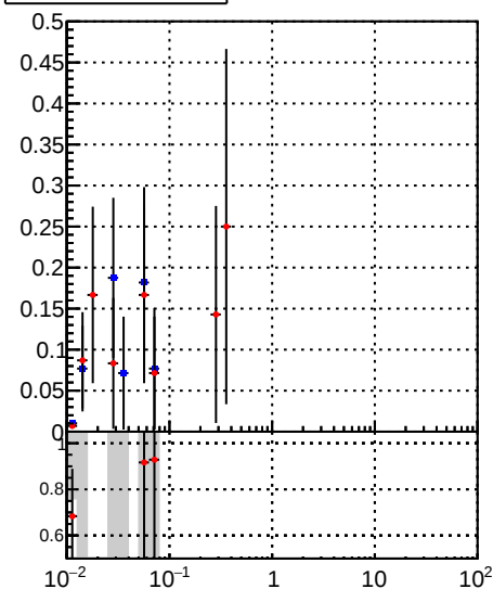
—●— DQM_DisplacedSUSY_mkFit_ —●— DQM_DisplacedSUSY_mkFit_BDT_
