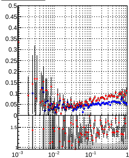
—•— DQM_DisplacedSUSY_mkFit_ —•— DQM_DisplacedSUSY_mkFit_BDT_
