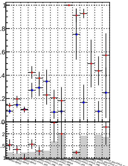
Fake rate vs. — DQM DisplacedSUSY mkFit — DQM DisplacedSUSY mkFit BDT
