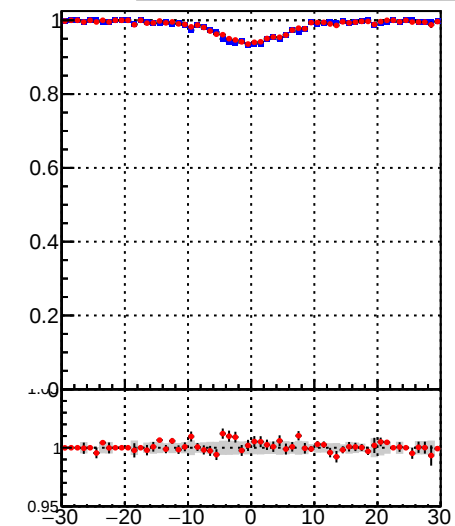
—•— DQM_DisplacedSUSY_mkFit_ —•— DQM_DisplacedSUSY_mkFit_BDT_
