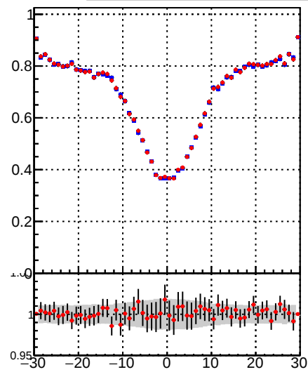
—•— DQM_DisplacedSUSY_mkFit_ —•— DQM_DisplacedSUSY_mkFit_BDT_
