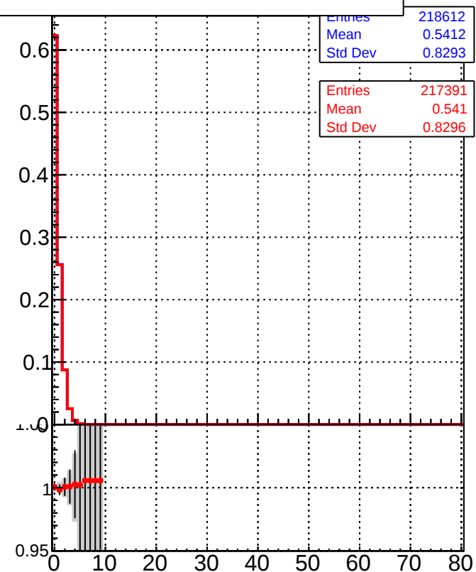
— DQM_DisplacedSUSY_mkFit_ — DQM_DisplacedSUSY_mkFit_BDT_
