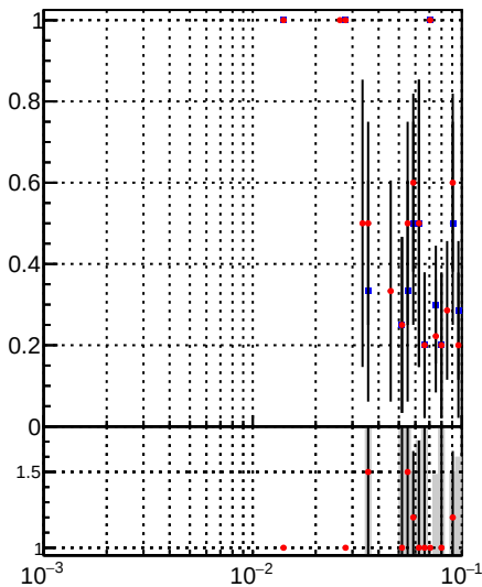
—•— DQM_DisplacedSUSY_mkFit_ —•— DQM_DisplacedSUSY_mkFit_BDT_
