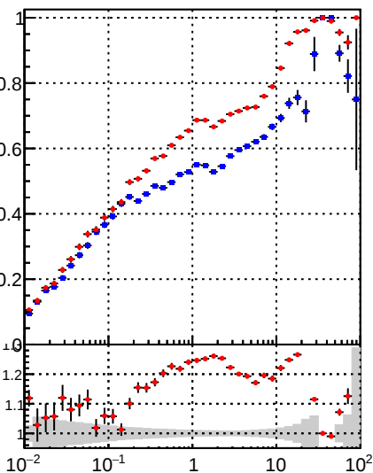
—•— DQM_DisplacedSUSY_mkFit_ —•— DQM_DisplacedSUSY_mkFit_BDT_
