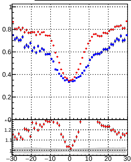
—•— DQM_DisplacedSUSY_mkFit_ —•— DQM_DisplacedSUSY_mkFit_BDT_
