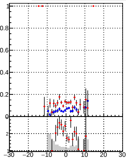
—•— DQM_DisplacedSUSY_mkFit_ —•— DQM_DisplacedSUSY_mkFit_BDT_
