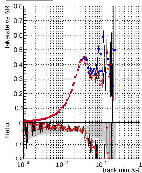
■ DQM_DisplacedSUSY_mkFit_ ■ DQM_DisplacedSUSY_mkFit_BDT_
