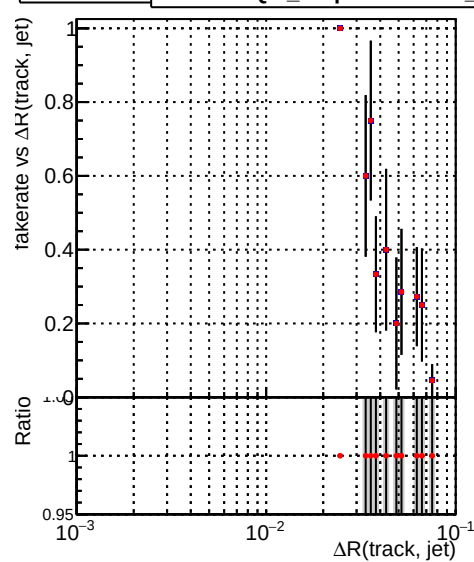
■ DQM_DisplacedSUSY_mkFit_ ■ DQM_DisplacedSUSY_mkFit_BDT_
