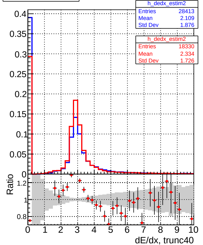
dE/dx estimator 2
