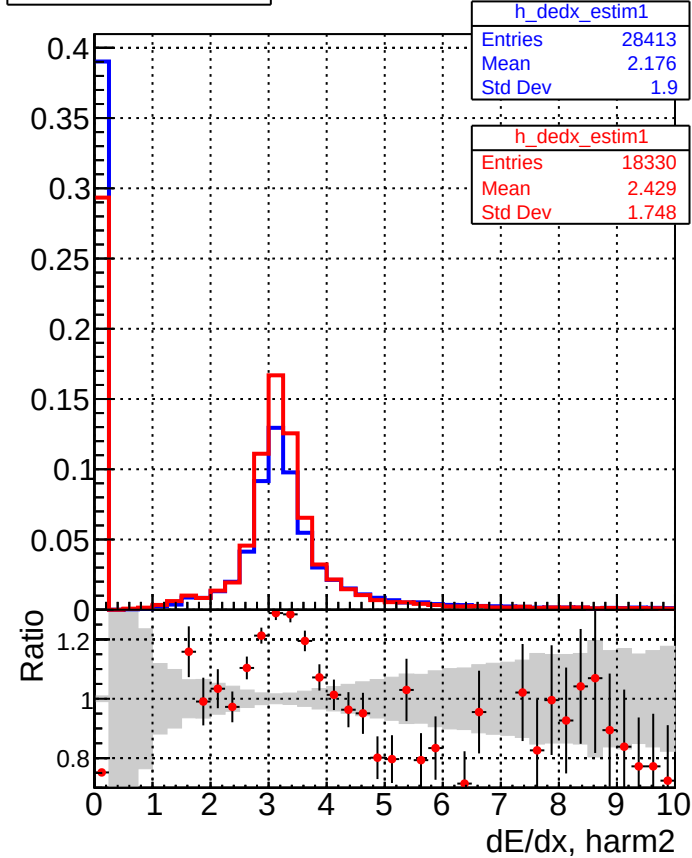
dE/dx estimator 1
