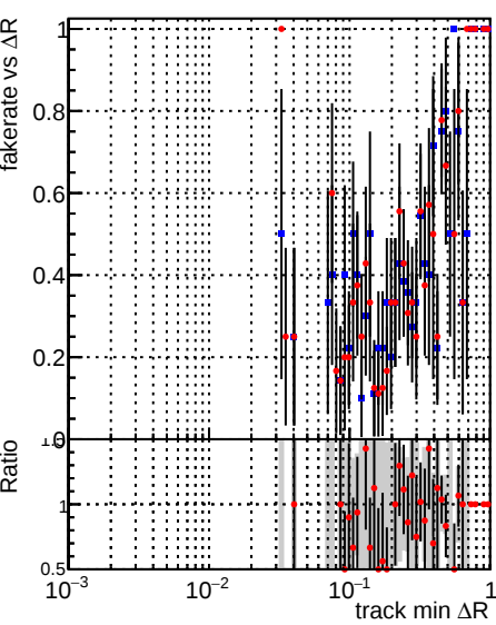
DQM_DisplacedSUSY_mkFit_ DQM_DisplacedSUSY_mkFit_BDT_
