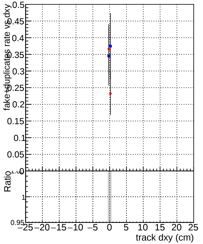
DQM_DisplacedSUSY_mkFit_ DQM_DisplacedSUSY_mkFit_BDT_
