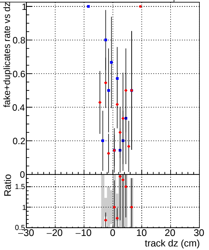
DQM_DisplacedSUSY_mkFit_ DQM_DisplacedSUSY_mkFit_BDT_
