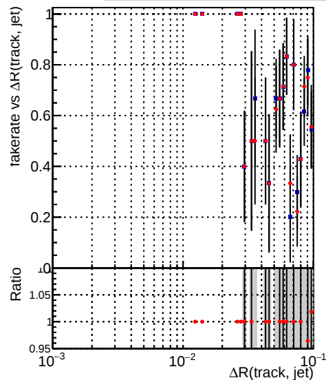
—•— DQM_DisplacedSUSY_mkFit_ —•— DQM_DisplacedSUSY_mkFit_BDT_
