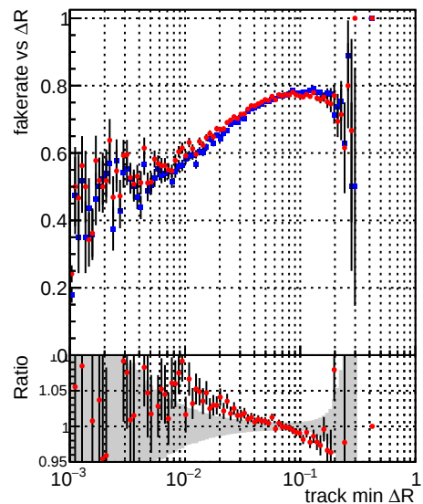
—•— DQM_DisplacedSUSY_mkFit_ —•— DQM_DisplacedSUSY_mkFit_BDT_
