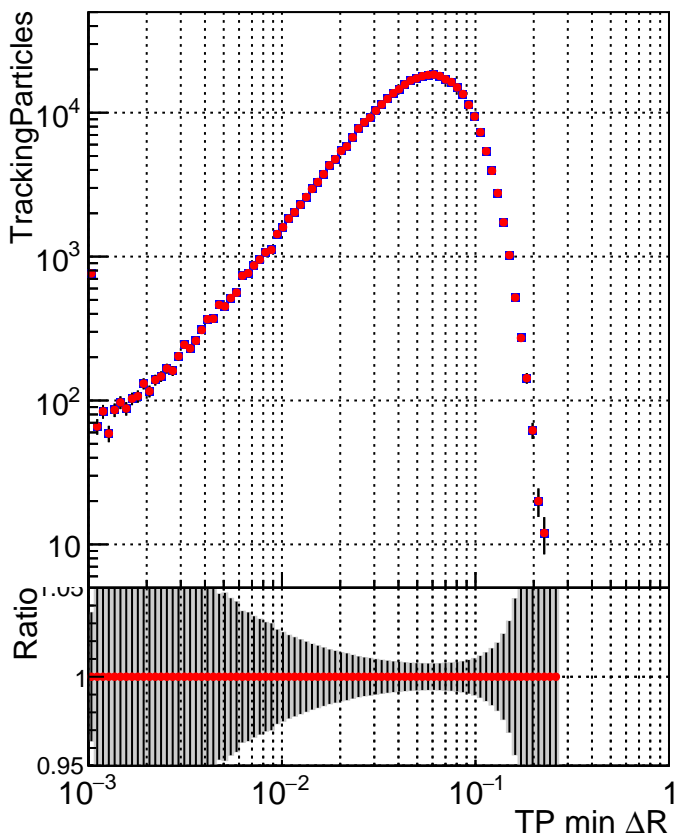
■ DQM_DisplacedSUSY_mkFit_ ■ DQM_DisplacedSUSY_mkFit_BDT_
