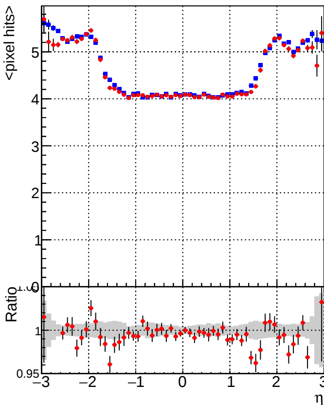
■ DQM_DisplacedSUSY_mkFit_ ● DQM_DisplacedSUSY_mkFit_BDT_
