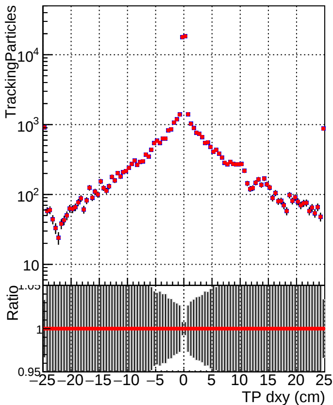
■ DQM_DisplacedSUSY_mkFit_ ● DQM_DisplacedSUSY_mkFit_BDT_
