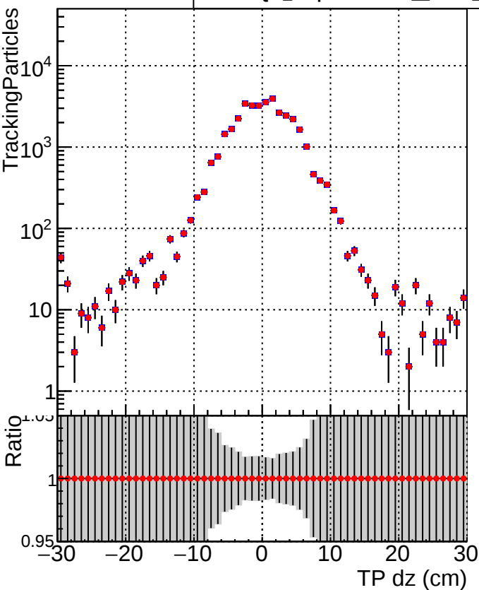
■ DQM_DisplacedSUSY_mkFit_ ● DQM_DisplacedSUSY_mkFit_BDT_
