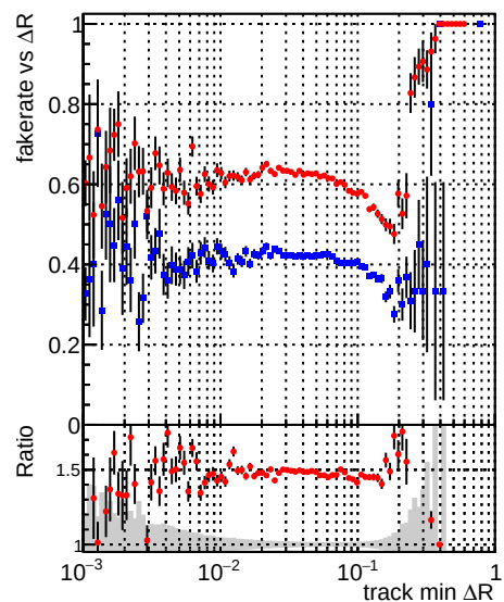
—●— DQM_DisplacedSUSY_mkFit_ —●— DQM_DisplacedSUSY_mkFit_BDT_
