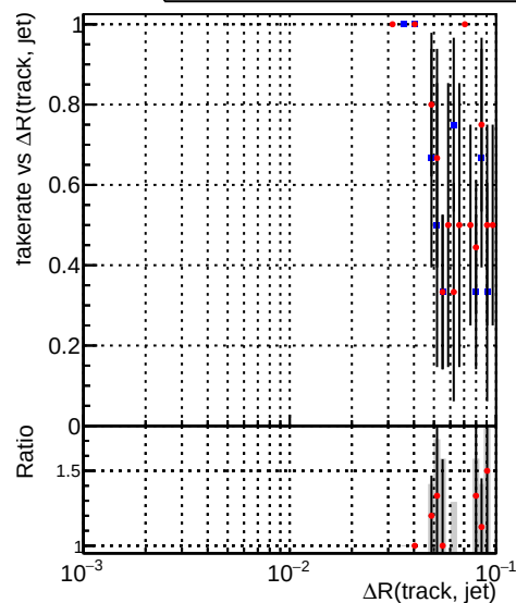
—●— DQM_DisplacedSUSY_mkFit_ —●— DQM_DisplacedSUSY_mkFit_BDT_
