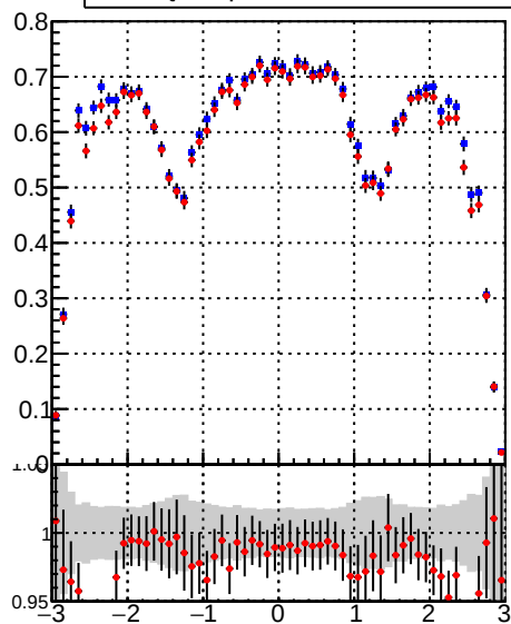
DQM_DisplacedSUSY_mkFit_ DQM_DisplacedSUSY_mkFit_BDT_
