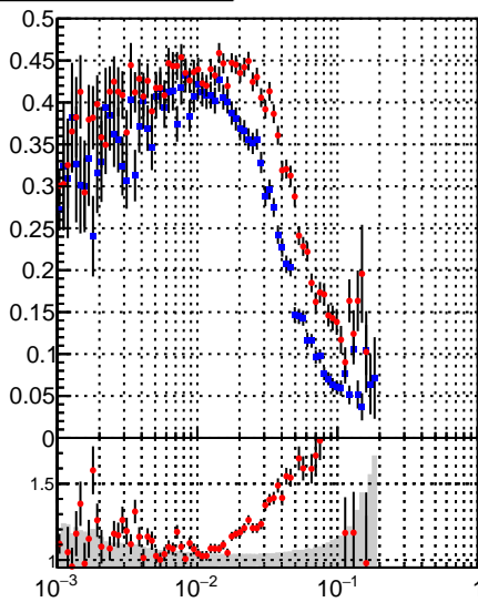
—●— DQM_DisplacedSUSY_mkFit_ —●— DQM_DisplacedSUSY_mkFit_BDT_
