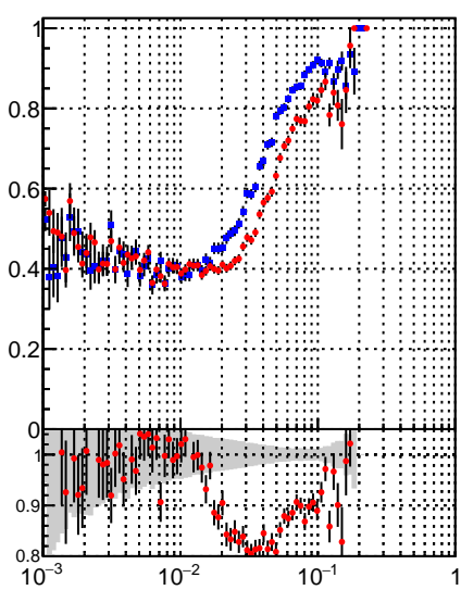
—●— DQM_DisplacedSUSY_mkFit_ —●— DQM_DisplacedSUSY_mkFit_BDT_
