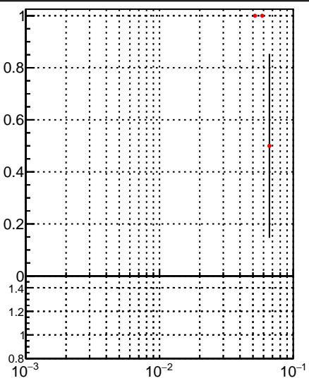
—●— DQM_DisplacedSUSY_mkFit_ —●— DQM_DisplacedSUSY_mkFit_BDT_
