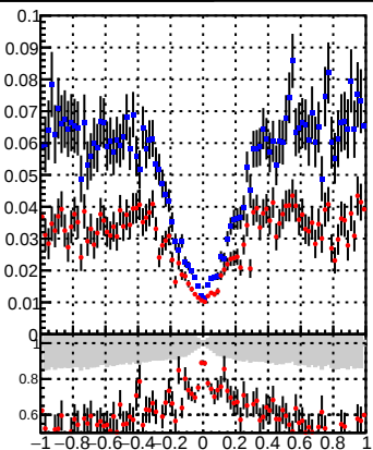
DQM_DisplacedSUSY_mkFit_
