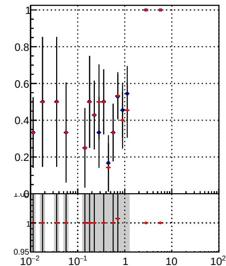
■ DQM_DisplacedSUSY_mkFit_ ■ DQM_DisplacedSUSY_mkFit_BDT_
