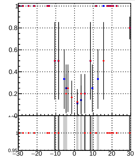
■ DQM_DisplacedSUSY_mkFit_ ■ DQM_DisplacedSUSY_mkFit_BDT_
