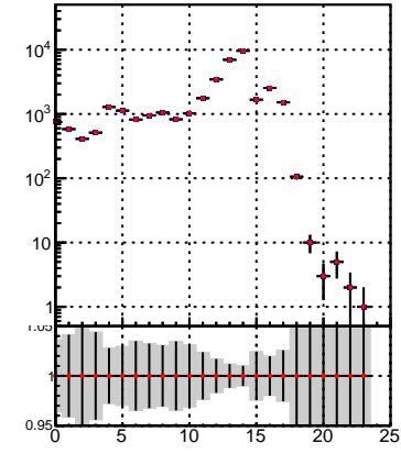
■ DQM_DisplacedSUSY_mkFit_ ■ DQM_DisplacedSUSY_mkFit_BDT_
