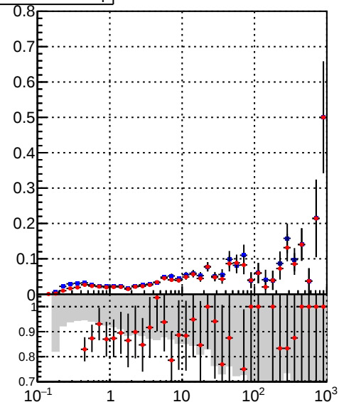
— DQM_DisplacedSUSY_mkFit_ — DQM_DisplacedSUSY_mkFit_BDT_
