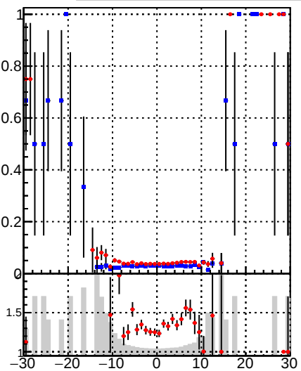
■ DQM_DisplacedSUSY_mkFit_ ■ DQM_DisplacedSUSY_mkFit_BDT_
