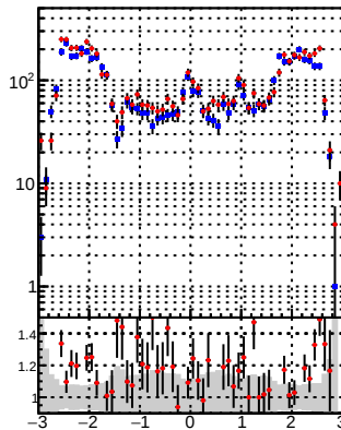
—●— DQM_DisplacedSUSY_mkFit —+— DQM_DisplacedSUSY_mkFit_BDT_
