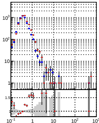
—●— DQM_DisplacedSUSY_mkFit —+— DQM_DisplacedSUSY_mkFit_BDT_
