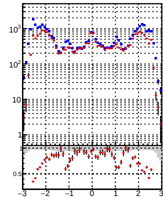
—●— DQM_DisplacedSUSY_mkFit —+— DQM_DisplacedSUSY_mkFit_BDT_
