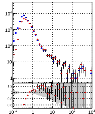
—●— DQM_DisplacedSUSY_mkFit —+— DQM_DisplacedSUSY_mkFit_BDT_
