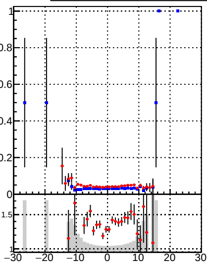
■ DQM_DisplacedSUSY_mkFit_ ● DQM_DisplacedSUSY_mkFit_BDT_
