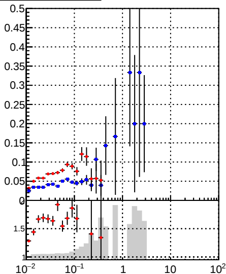
■ DQM_DisplacedSUSY_mkFit_ ● DQM_DisplacedSUSY_mkFit_BDT_
