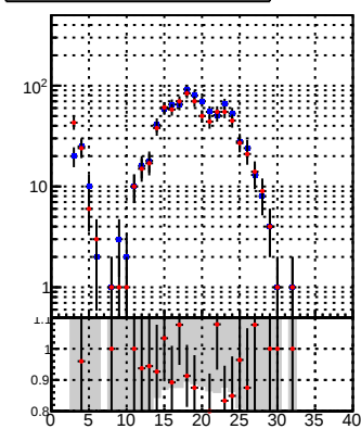
—●— DQM_DisplacedSUSY_mkFit_ —●— DQM_DisplacedSUSY_mkFit_BDT_
