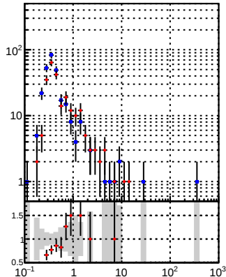
—●— DQM_DisplacedSUSY_mkFit —×— DQM_DisplacedSUSY_mkFit_BDT_
