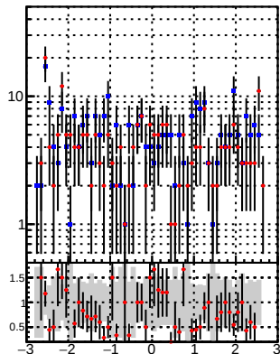
—●— DQM_DisplacedSUSY_mkFit —×— DQM_DisplacedSUSY_mkFit_BDT_
