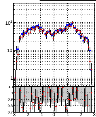
N of reco track vs ps eta
