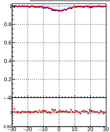
—•— DQM_DisplacedSUSY_mkFit_ —•— DQM_DisplacedSUSY_mkFit_BDT_
