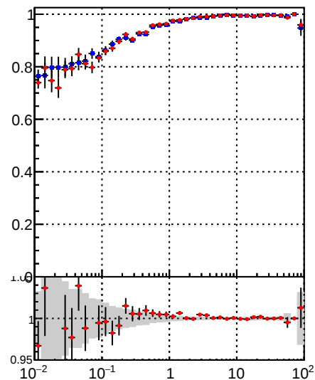
—•— DQM_DisplacedSUSY_mkFit_ —•— DQM_DisplacedSUSY_mkFit_BDT_
