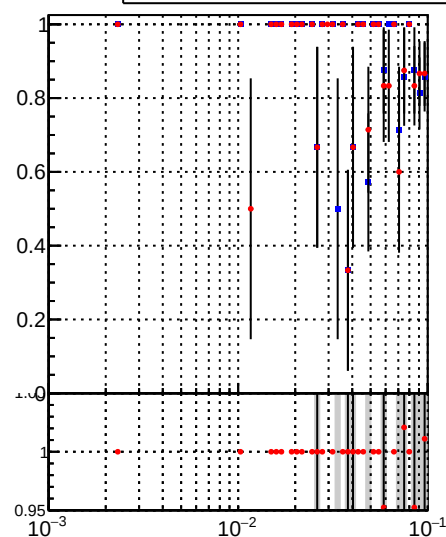
—•— DQM_DisplacedSUSY_mkFit_ —•— DQM_DisplacedSUSY_mkFit_BDT_
