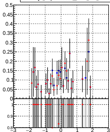
■ DQM_DisplacedSUSY_mkFit_ ■ DQM_DisplacedSUSY_mkFit_BDT_
