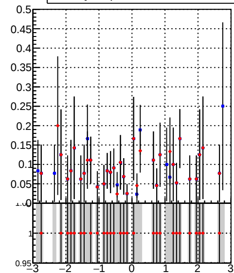
DQM_DisplacedSUSY_mkFit_ DQM_DisplacedSUSY_mkFit_BDT_
