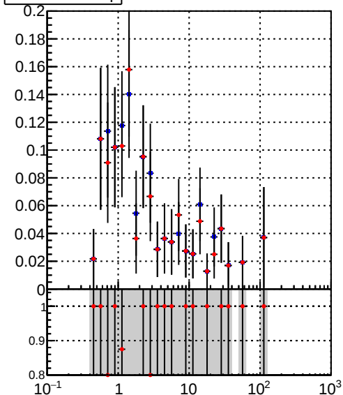
DQM_DisplacedSUSY_mkFit_ DQM_DisplacedSUSY_mkFit_BDT_
