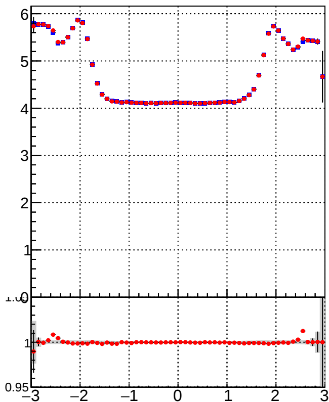
■ DQM_DisplacedSUSY_mkFit_ ● DQM_DisplacedSUSY_mkFit_BDT_
