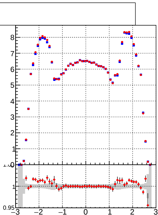
■ DQM_DisplacedSUSY_mkFit_ ● DQM_DisplacedSUSY_mkFit_BDT_
