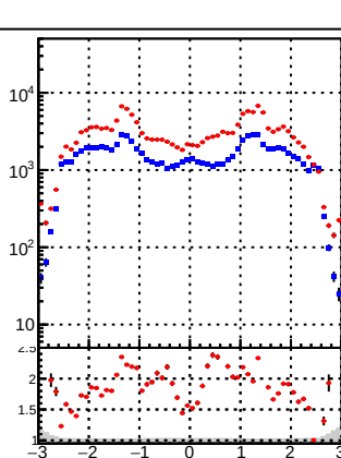
—●— DQM_DisplacedSUSY_mkFit —×— DQM_DisplacedSUSY_mkFit_BDT
